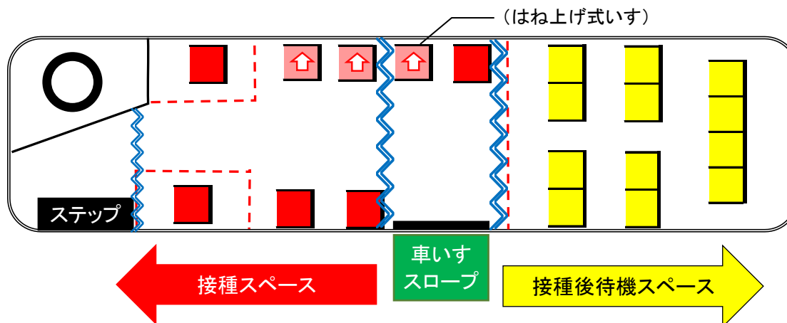
中型路線バス(車長9m ノンステップ車)
