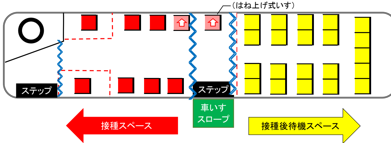
大型路線バス(車長11m ワンステップ車)
